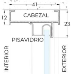
5 CORTE VERTICAL CABEZAL
